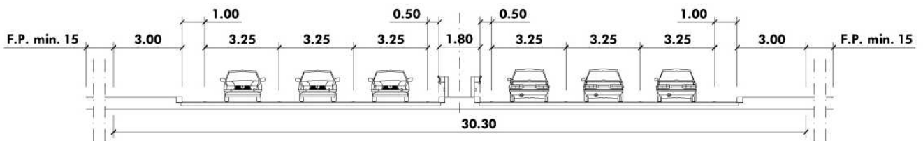
SOLUZIONE A 3+3 CORSIE DI MARCIA
