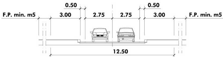
SOLUZIONE BASE A 1 + 1 CORSIE DI MARCIA
