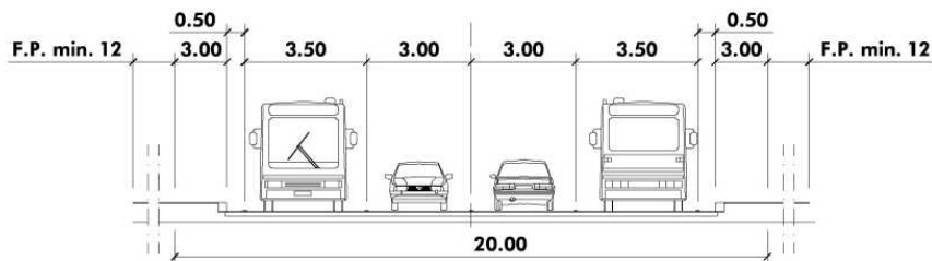
SOLUZIONE A 2 + 2 CORSIE DI MARCIA DI CUI 1 + 1 PERCORSE DA AUTOBUS (in ambito scarsamente edificato e con modesto traffico pedonale)
