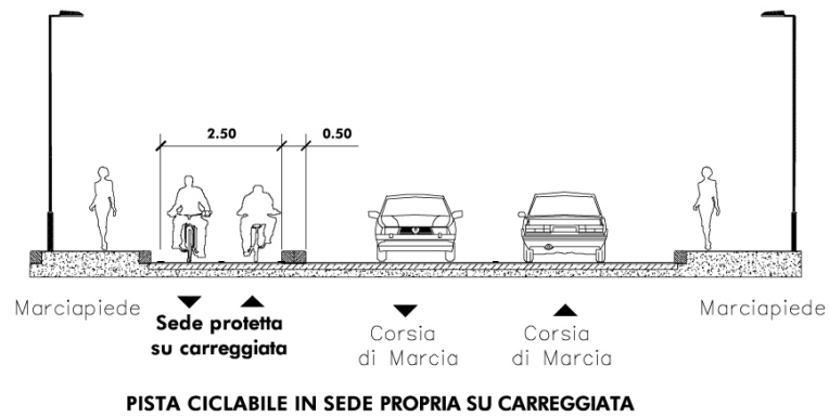
FIGURA 8.1 Ubicazione delle piste ciclabili sulle sedi stradali
