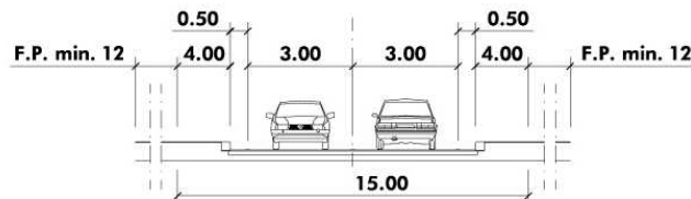
SOLUZIONE BASE A 1+1 CORSIE DI MARCIA (scarso traffico pesante)
