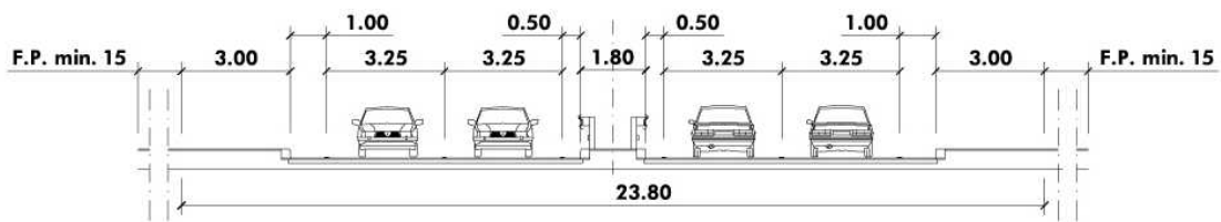
SOLUZIONE BASE A 2+2 CORSIE DI MARCIA
