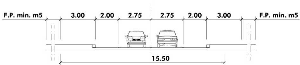
SOLUZIONE A 2 CORSIE DI MARCIA CON DUE FILE DI STALLI DI SOSTA IN LINEA
