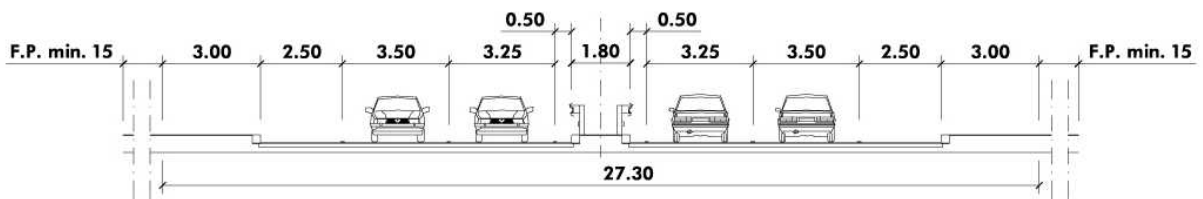
SOLUZIONE A 2+2 CORSIE DI MARCIA CON CORSIA DI EMERGENZA (PRESENZA DI TRAFFICO PESANTE)
