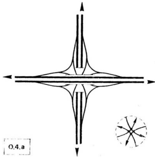
SVINCOLO A STELLA A 3 LIVELLI (il livello intermedio a raso per le svolte a sinistra può eventualmente essere semaforizzato)
