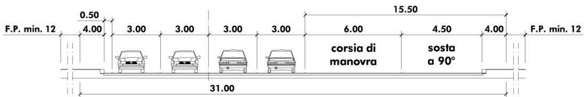
SOLUZIONE BASE A 2+2 CORSIE DI MARCIA (con presenza di sosta e scarso traffico pesante)
