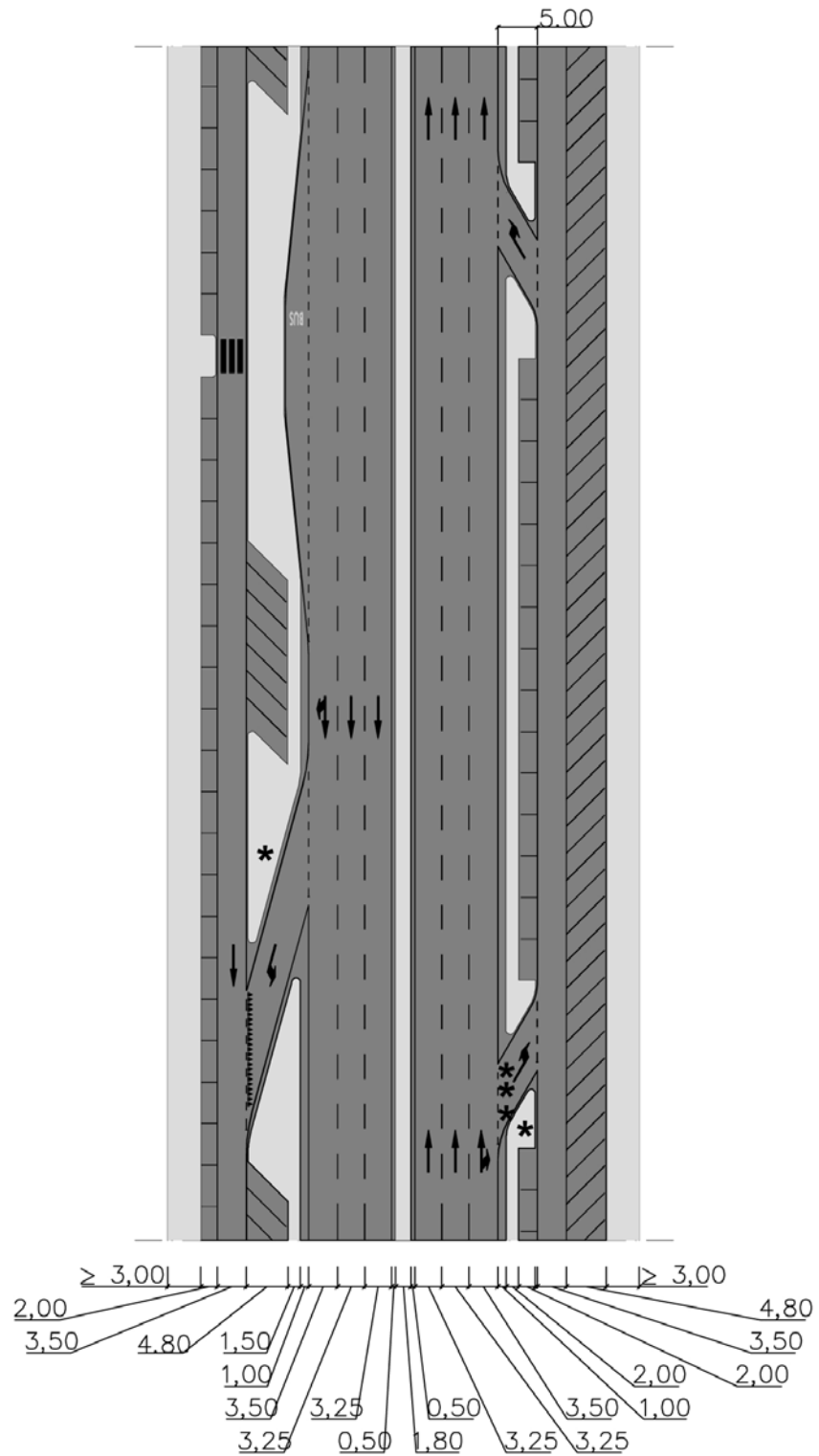
FIGURA 8.3 schemi esemplificativi di parcheggi su strada: aree di sosta separate dalla carreggiata (strada di scorrimento)
